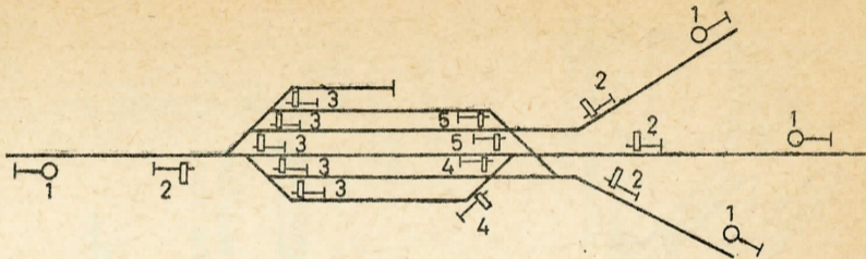
188. ábra. Alakjelzők elhelyezése állomásokon
